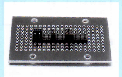
ジャンプソケット (JS-1) (60ページ参照) (WLW-1とJS-1の組合せ)
