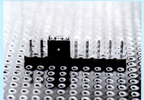
ジャンプソケット (JS-1) (60ページ参照) を使用した場合 (WL-1とJS-1の組合せ)
