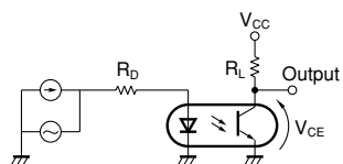
Fig.16 周波数特性の測定回路
