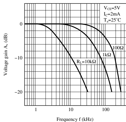
Fig.15 周波数特性
