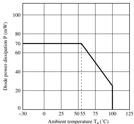
Fig.4 全許容損失低減曲線
