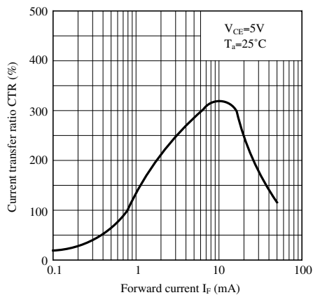
Fig.6 電流伝達比—順電流特性
