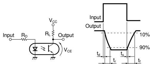
Fig.14 応答時間の測定回路
