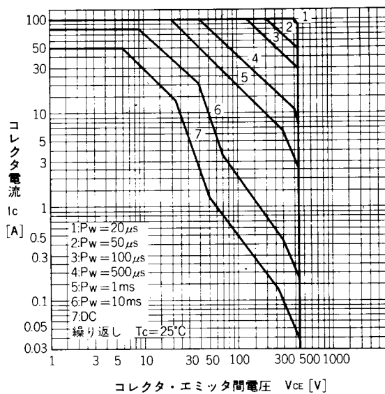
安全動作領域特性 Safe Operating Area
